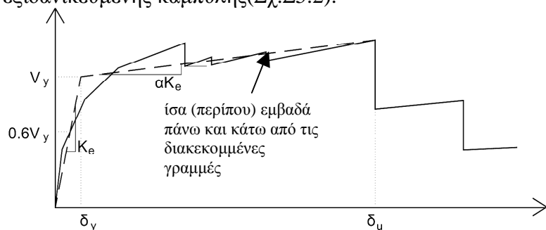
Σχ. Σ5.2 Εξιδανίκευση μιας (σημασιακής) καμπύλης αντίστασης της κατασκευής με διγραμμική καμπύλη
