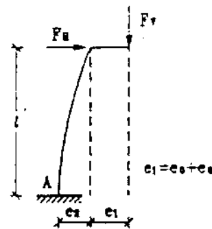
Σχήμα 14.3 Πρότυπο υποστυλώμα
